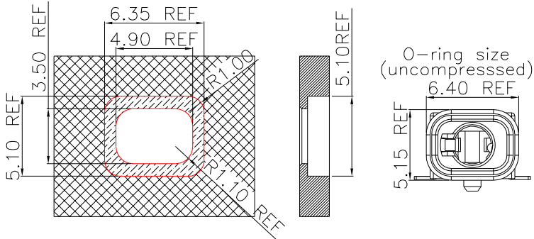
面板开孔参考尺寸
