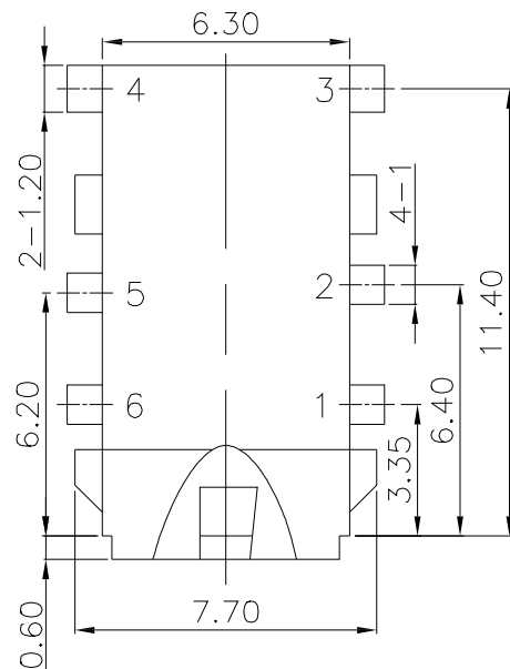
P.C.B LAYOUT
