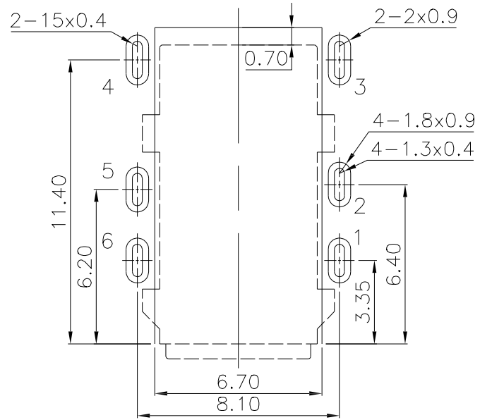
P.C.B LAYOUT
