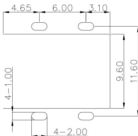
P.C.B LAYOUT
